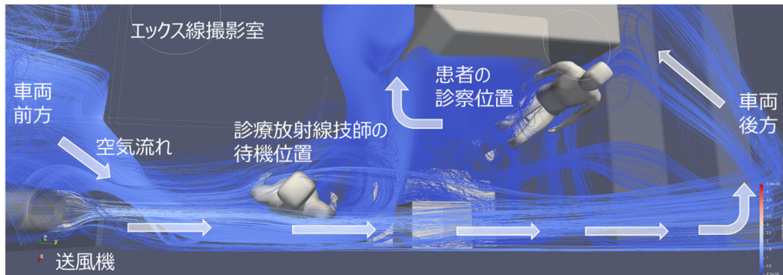
図 3 車内気流の数値シミュレーションの一例
